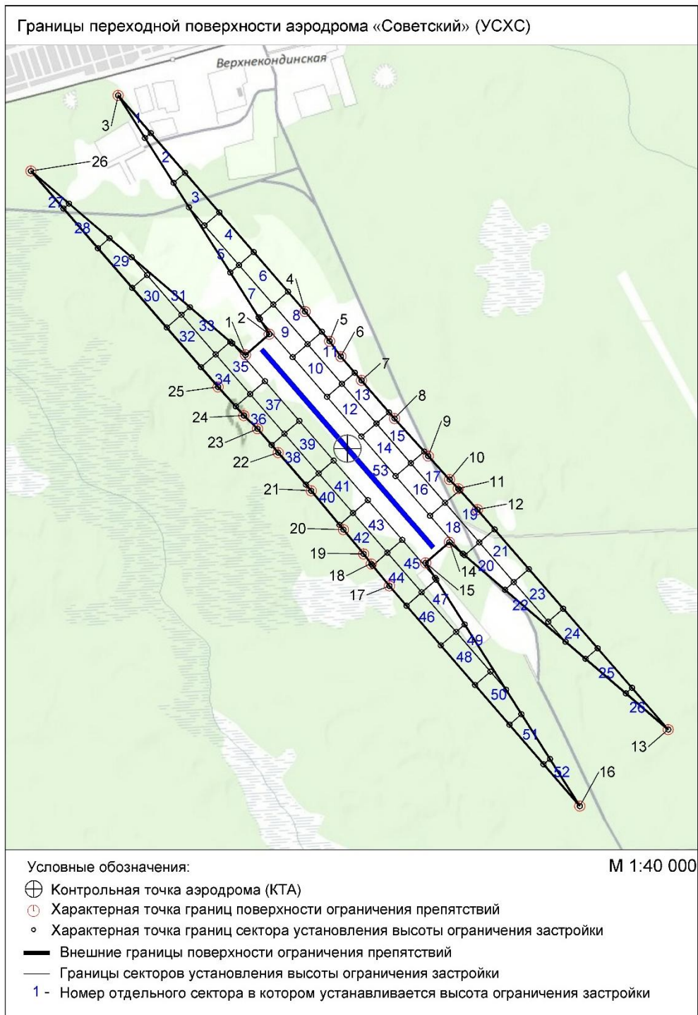
Рисунок 4.2. Схема границ переходной поверхности с учетом летной полосы для ВПП 12/30
