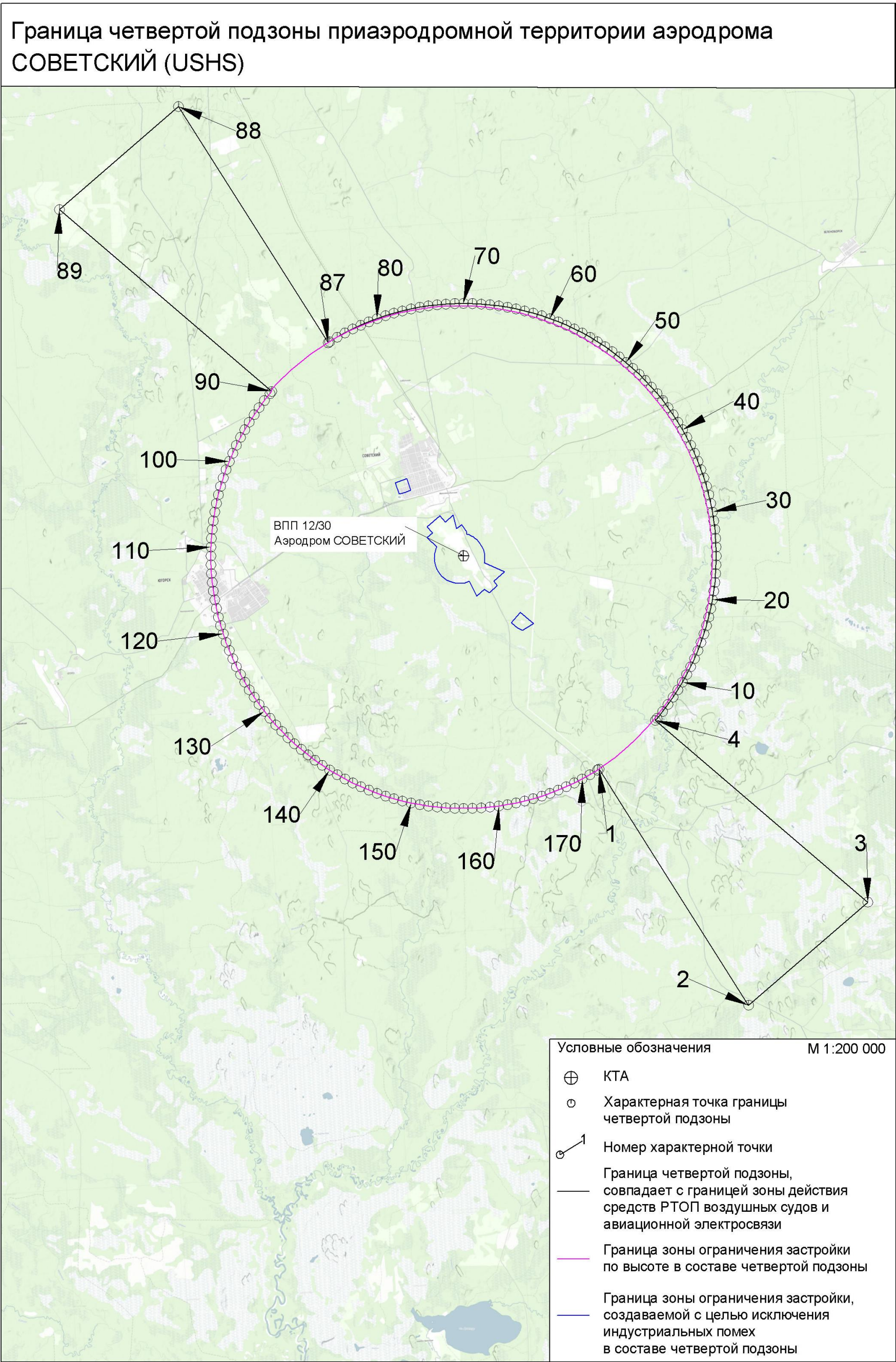
Рисунок 5.1. Схема границ четвертой подзоны
