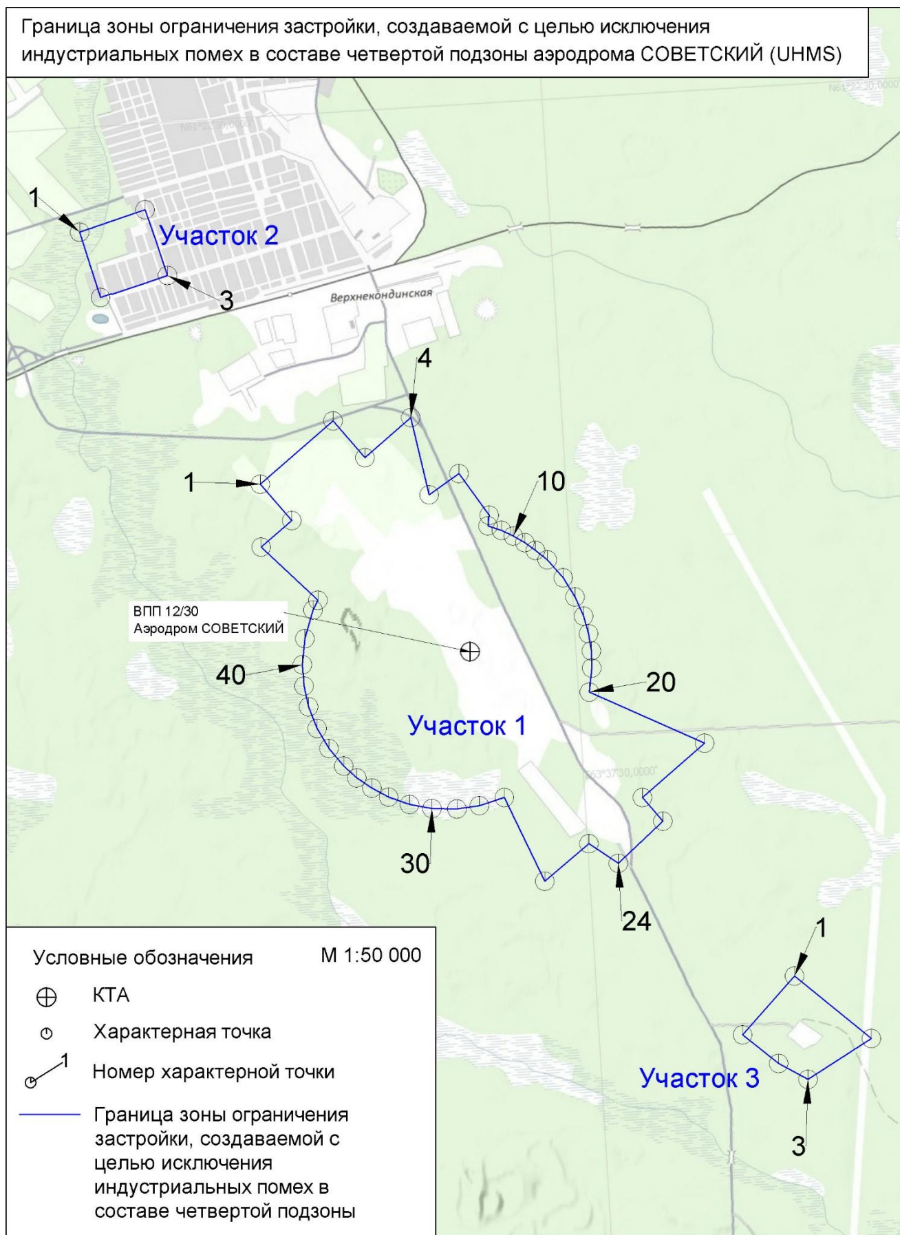
Рисунок 5.2. Схема границы зоны ограничения застройки, создаваемой с целью исключения индустриальных помех в составе четвертой подзоны приаэродромной территории
